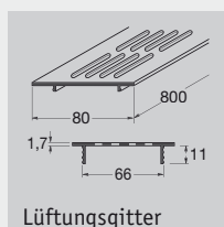
Lüftungsgitter
